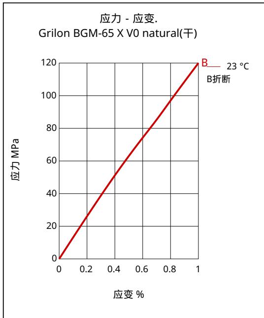
应力 - 应变.
